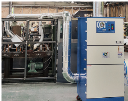
스릴거꾸집생산 - 40CMM
