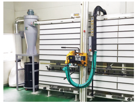
아크릴절단 - 40CMM
